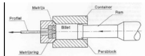
figuur 2: schematische voorstelling van het extrusieproces.
